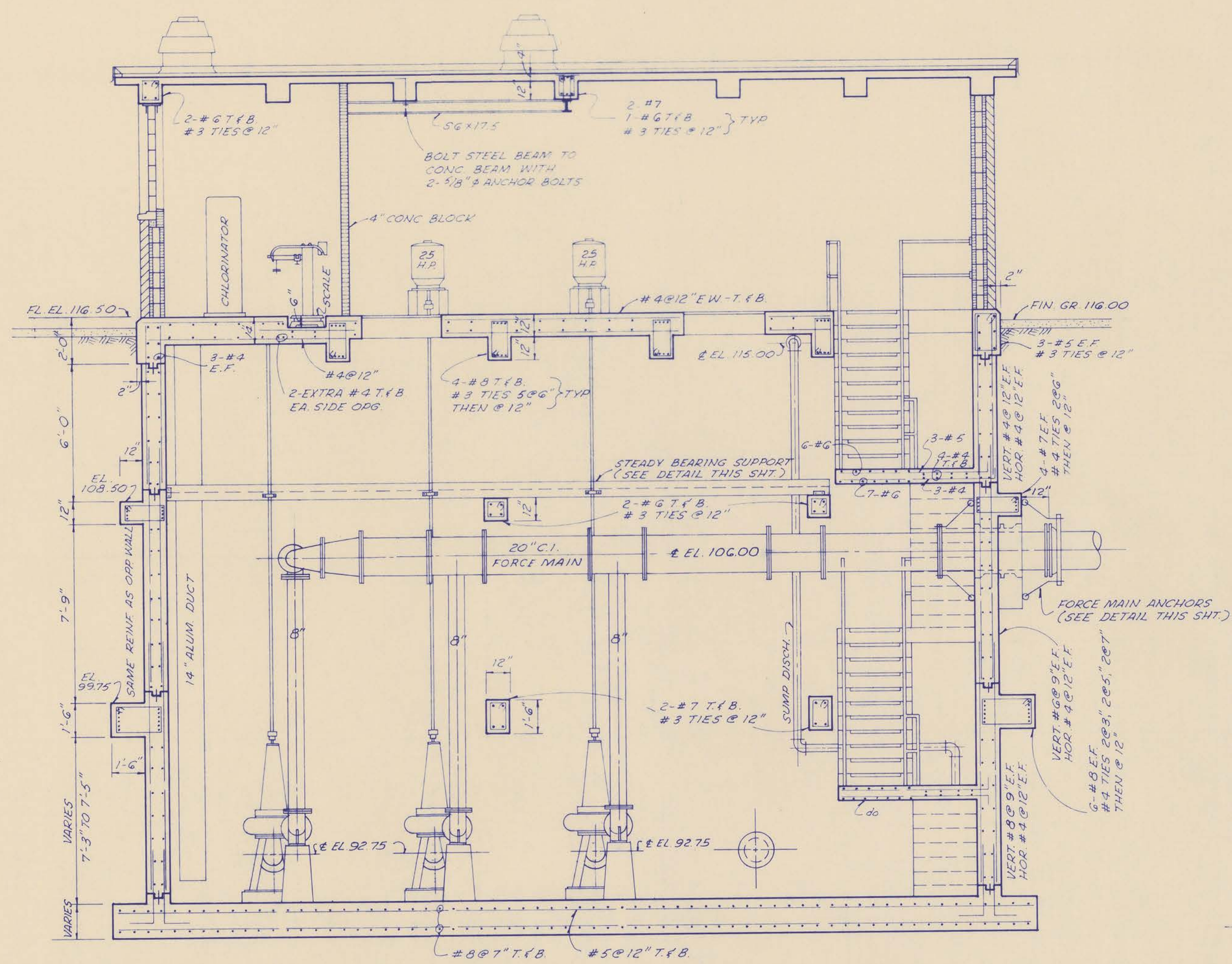
SECTION A-A 1/4"=1'-0"
