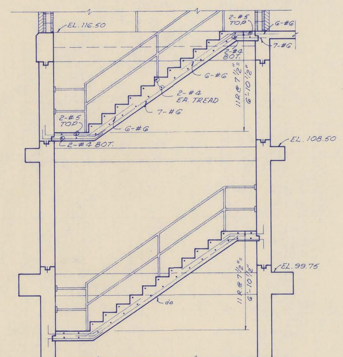
SECTION D-D 1/4"=1'-0"
